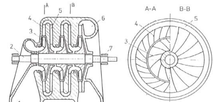
Řez třístupňovým radiálním turbokompresorem
